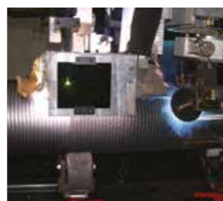
Recubrimiento a 360 grados para tuberías/colectores
