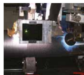
Revestimento orbital de tubo coletor
