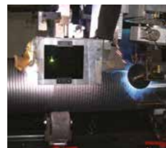
Rechargement par soudage à 360° de tubes ou de collecteurs
