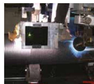
Saldatura su tubo 360/ rivestimento collettore
