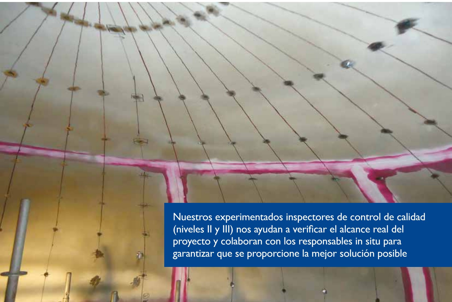
Inspección por líquidos penetrantes
