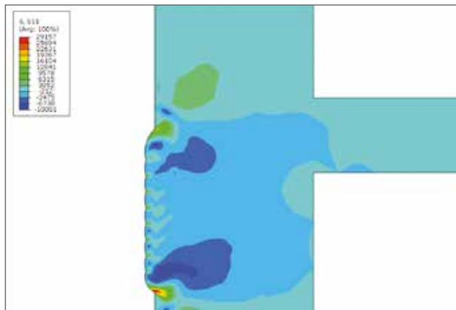
Predicción de la tensión residual radial
