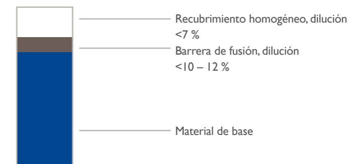
Ilustración esquemática de una sección transversal
