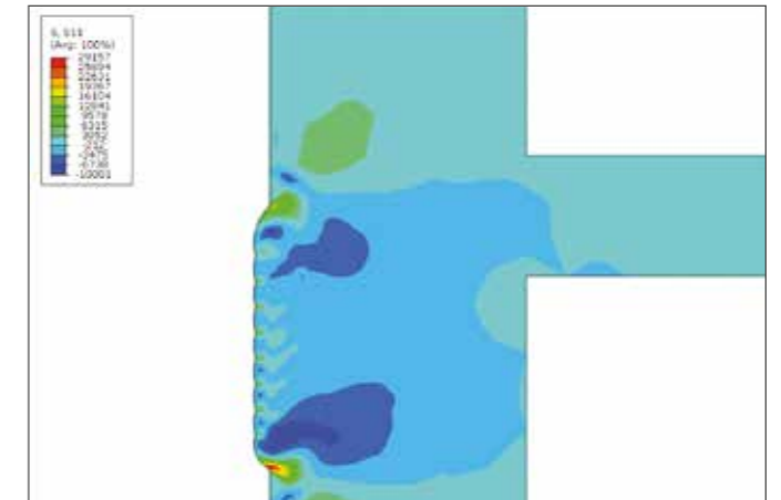
Predicción de la tensión residual radial
