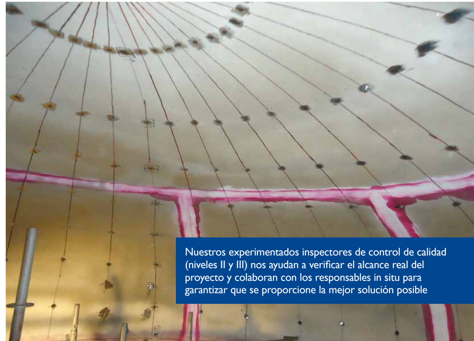
Inspección por líquidos penetrantes
