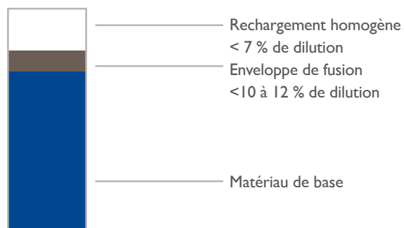
Représentation schématique d’une section transversale
